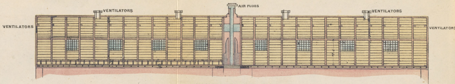
LONGITUDINAL SECTION C
